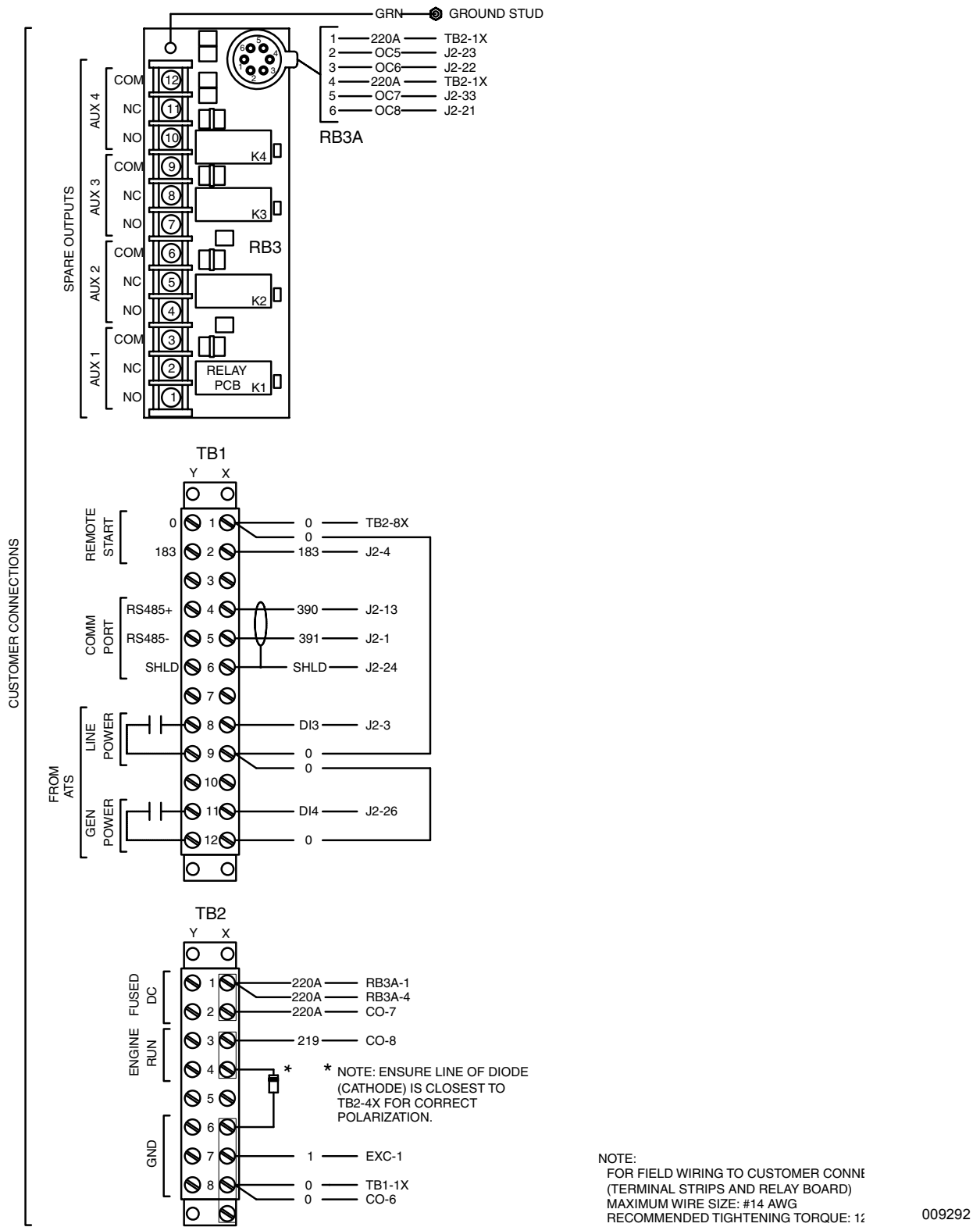
Рис. 8-3. Схема типовой промышленной панели соединений низкого напряжения
