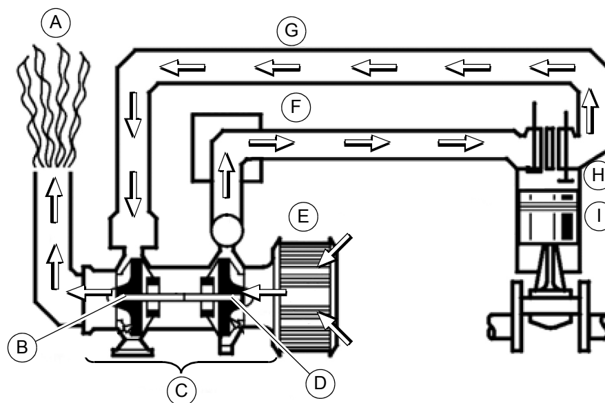
Рис. 5-1. Работа турбонагнетателя
