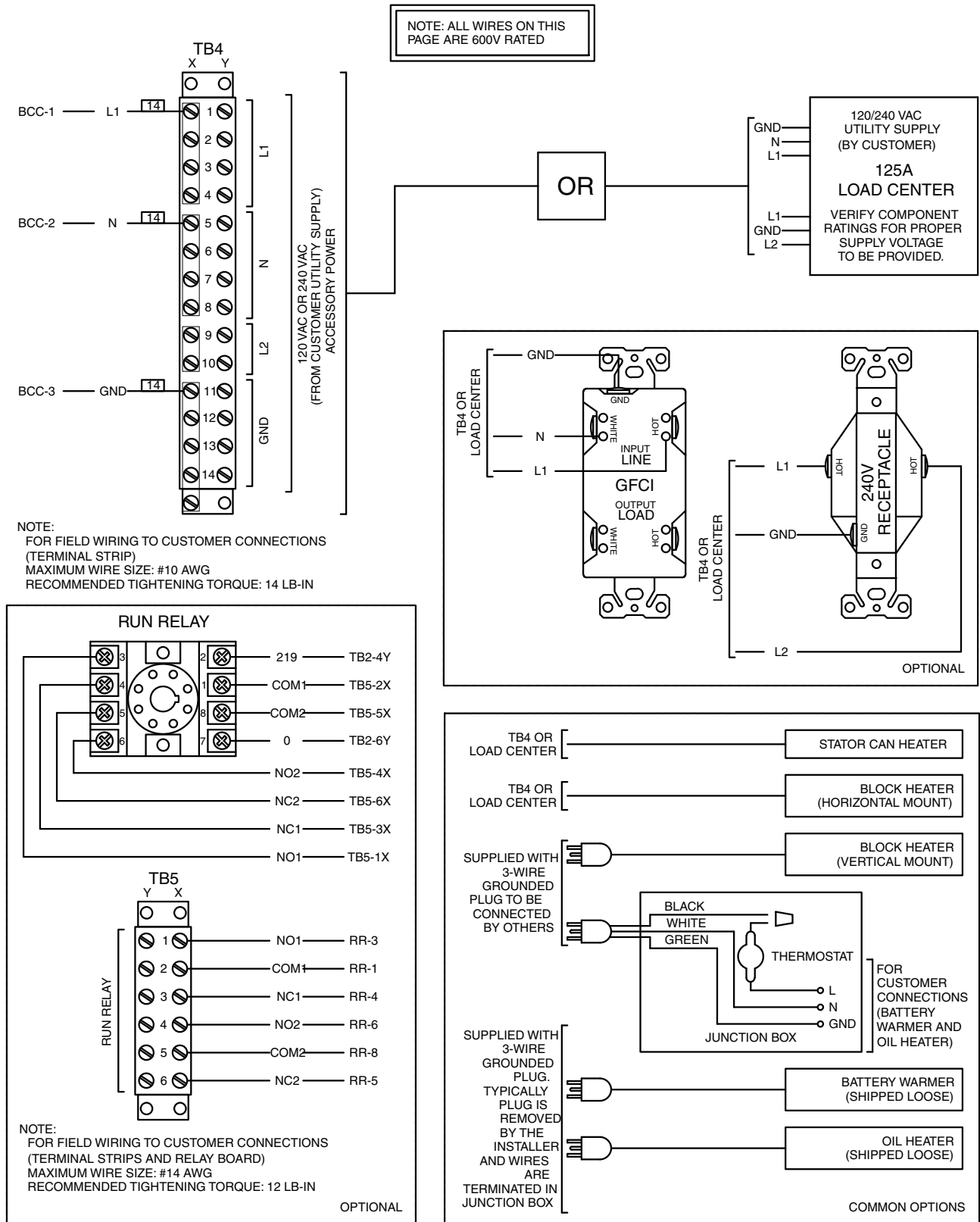
Рис. 8-2. Типовые соединения заказчика в модуле соединений высокого напряжения
