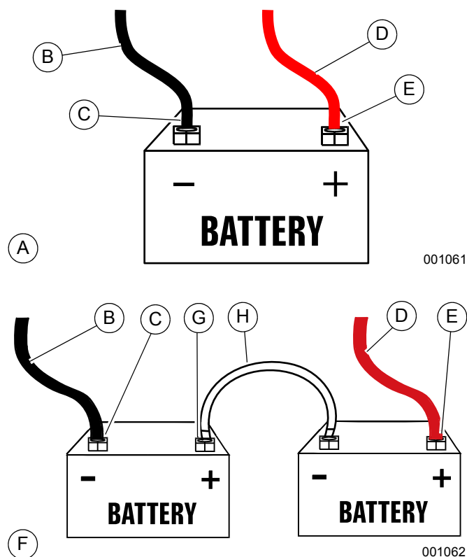
Рис. 8-4. Соединения кабелей батареи
