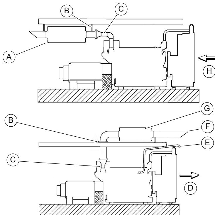
Рис. 5-11. Внутренний и наружный глушитель
