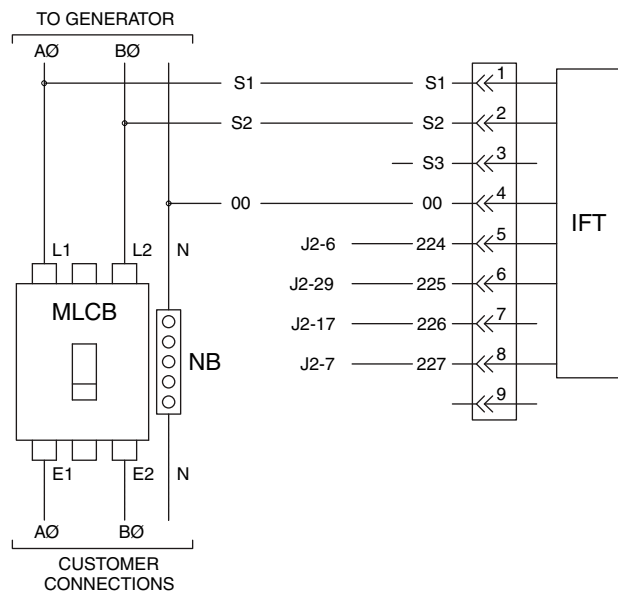
Рис. 8-1. Типовая промышленная схема, показывающая соединения проводов нагрузки с главным автоматическим выключателем
