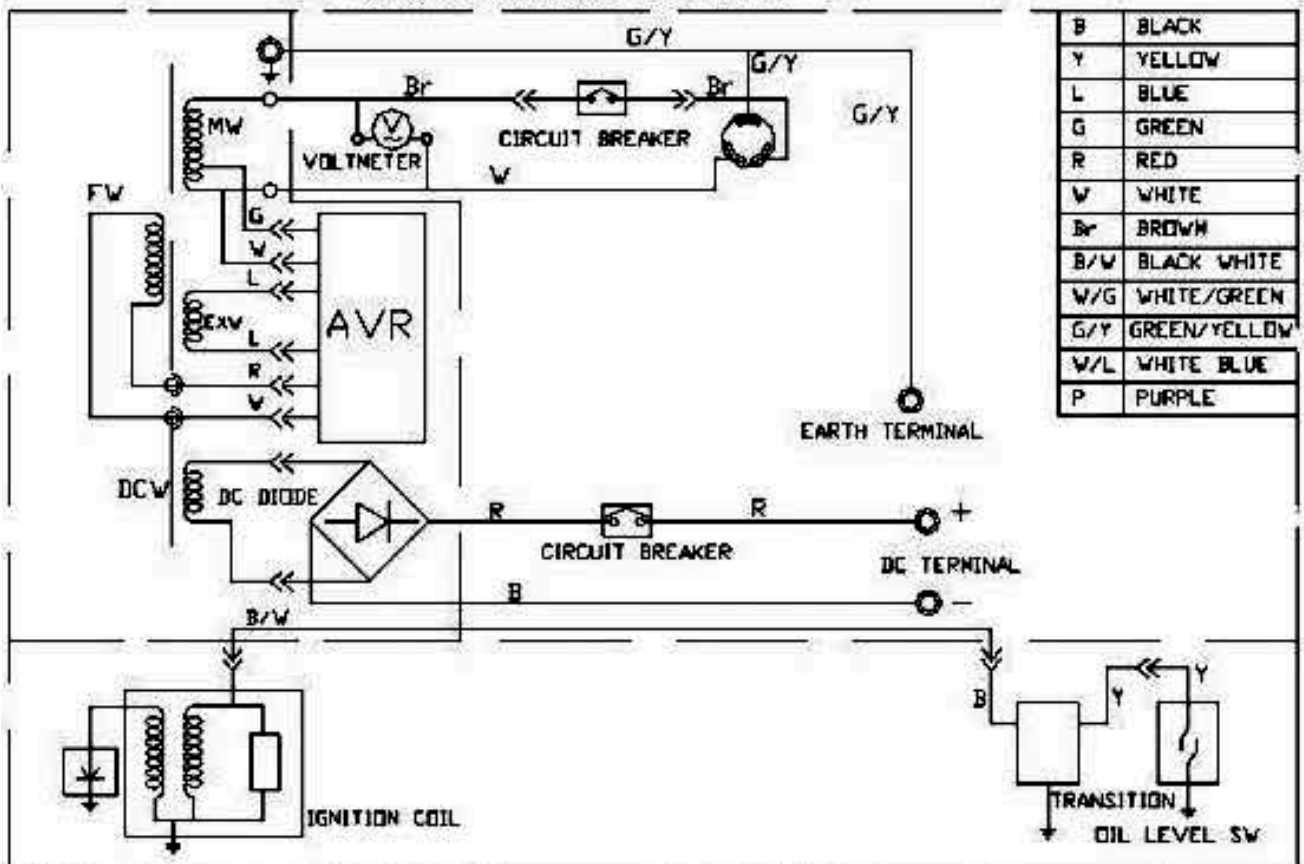
CC1500-G-B 220V/50Hz 燃气发电机组电路图
