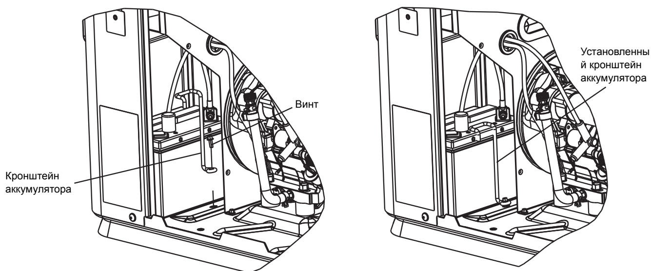
Рис. 4-7. Установка аккумулятора
