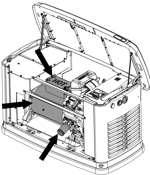
Рис. 1-2. Горячие поверхности
